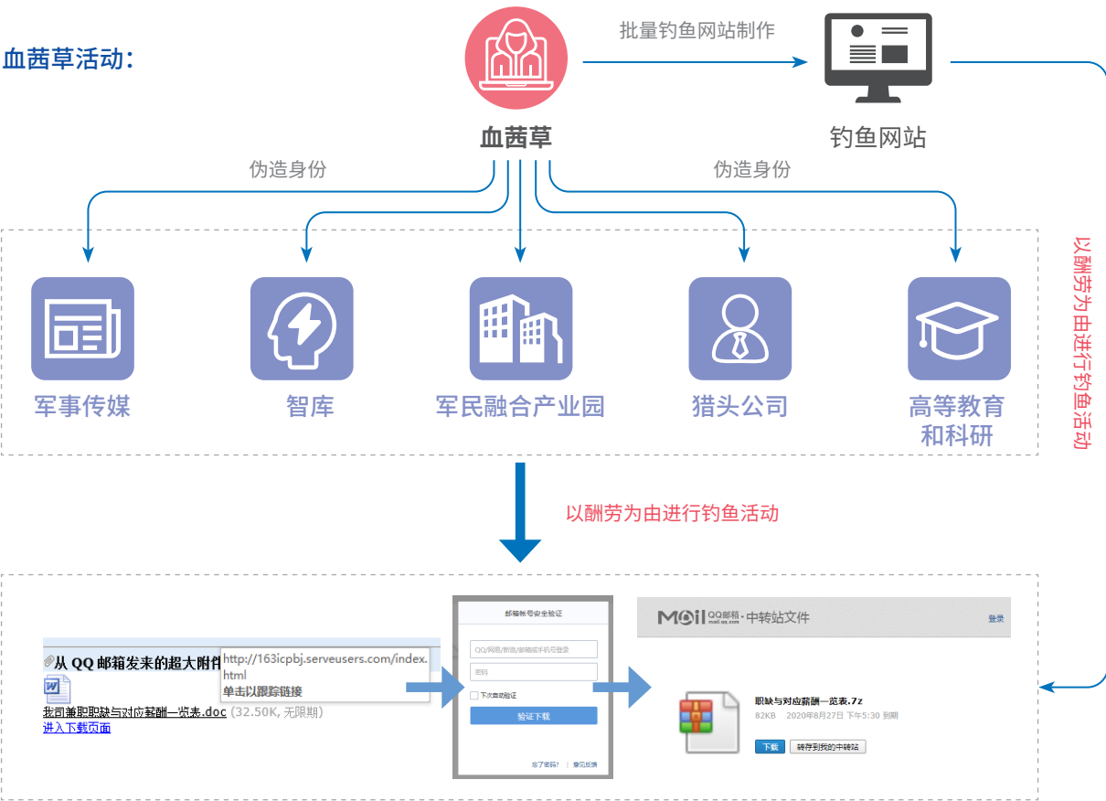
▲ 图 3.3 血茜草活动常用攻击手法
